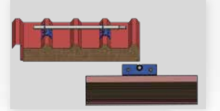
Çatı Paneli - Trapez Uyumlu Tek Borulu Kar Tutucu
