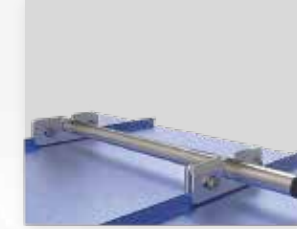
180° Kenet Tek Borulu Kar Tutucu Sistem
