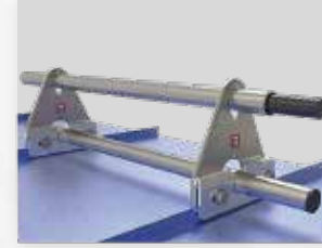
180° Kenet Çift Borulu Kar Tutucu Sistem
